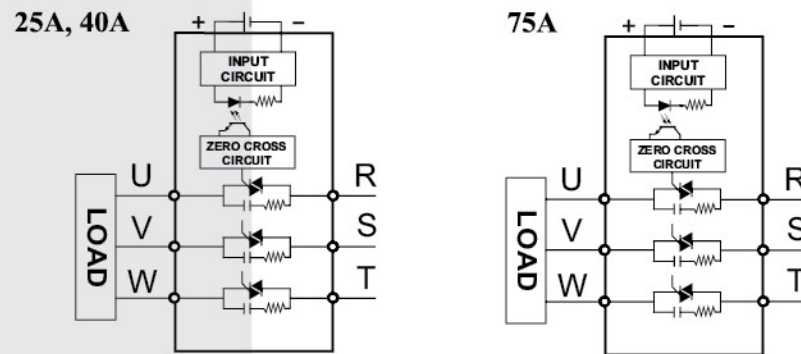
Схемы подключения
