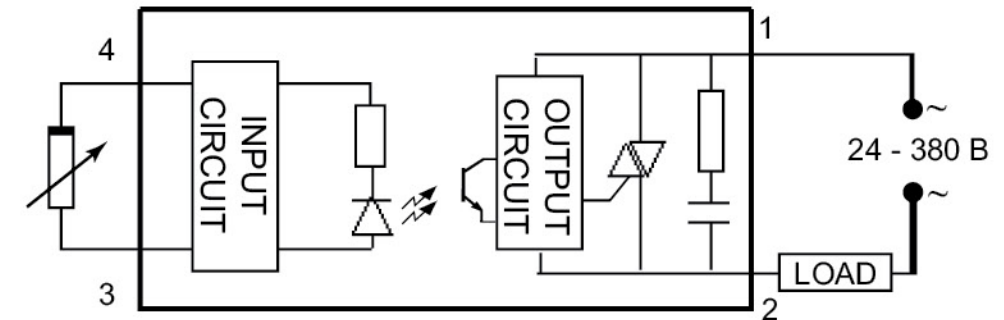
Схема подключения
