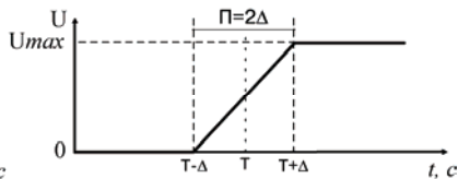
б) прямо-пропорциональное регулирование
