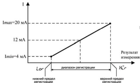
Рисунок 3.7 – Принцип формирования выходного сигнала ВУ в режиме регистратора для приборов с ВУ типа И
